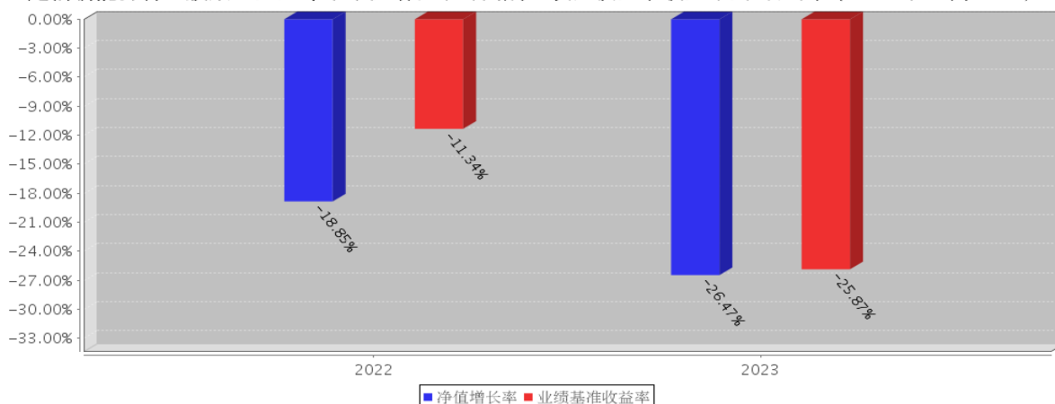
建信新能源行业股票C 基金每年净值增长率与同期业绩比较基准收益率的对比图 (2023年12月31日)
